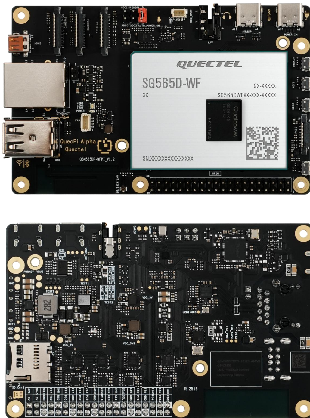
图 5：俯视图和底视图
