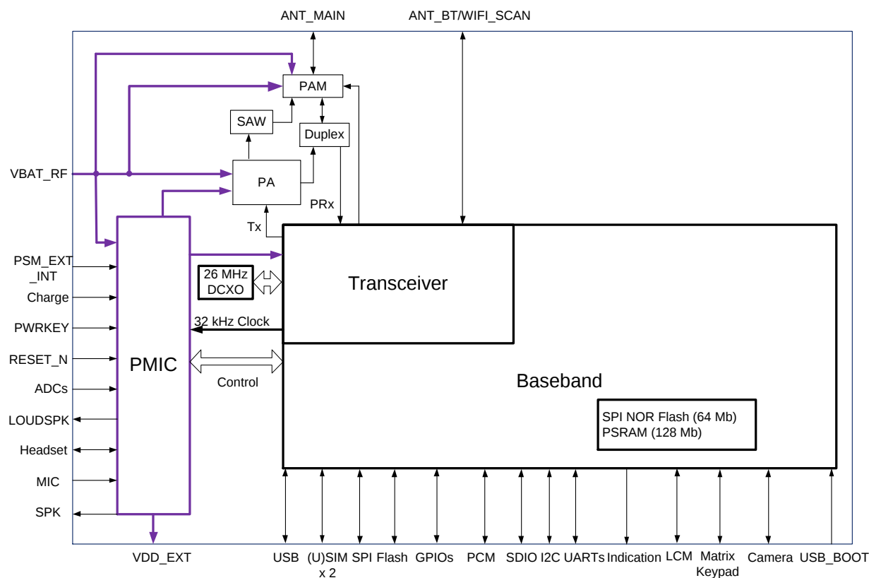
图 1: 功能框图
