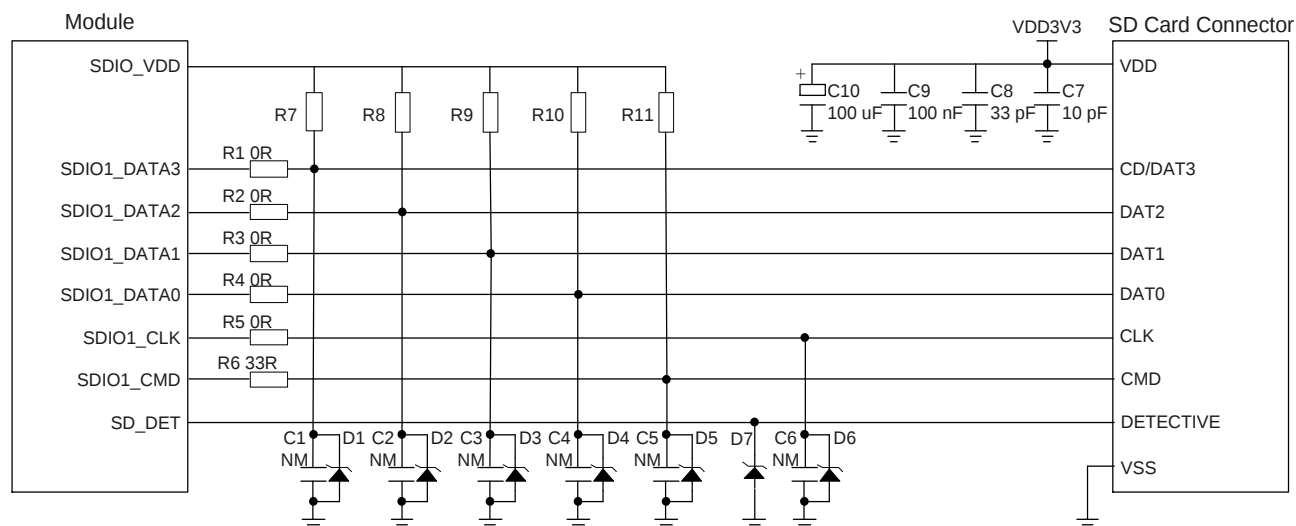
图 31: SD 卡接口电路参考设计
