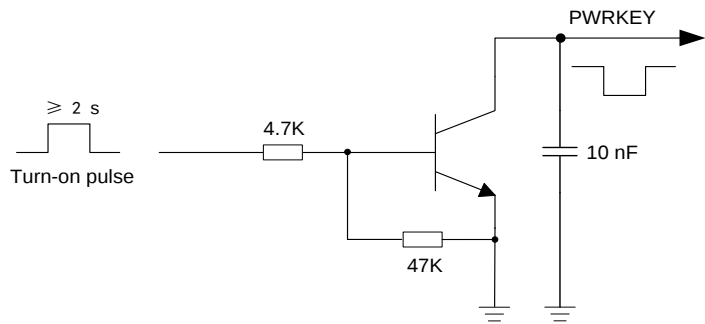
图 12: 开集驱动开机参考电路
