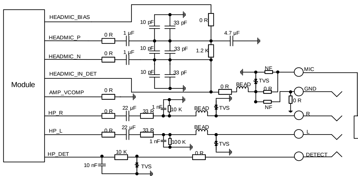
图 30：耳机接口参考电路
