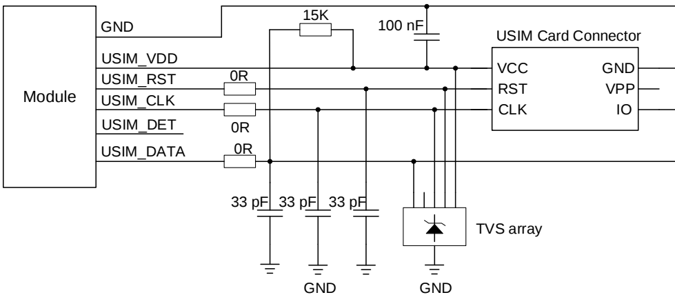
图 21: 6-pin (U)SIM 接口参考电路图
