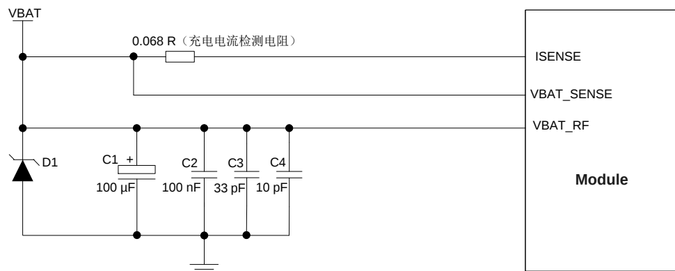
图 10：模块供电电路（带充电功能）
