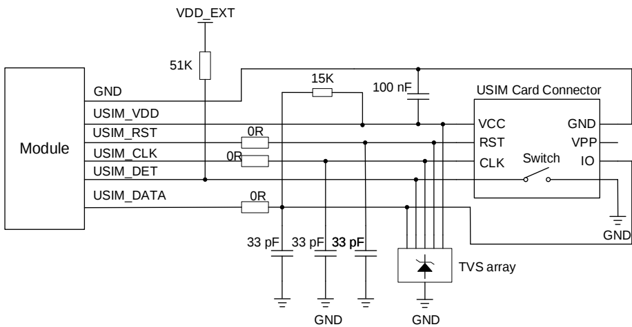
图 20: 8-pin (U)SIM 接口参考电路图
