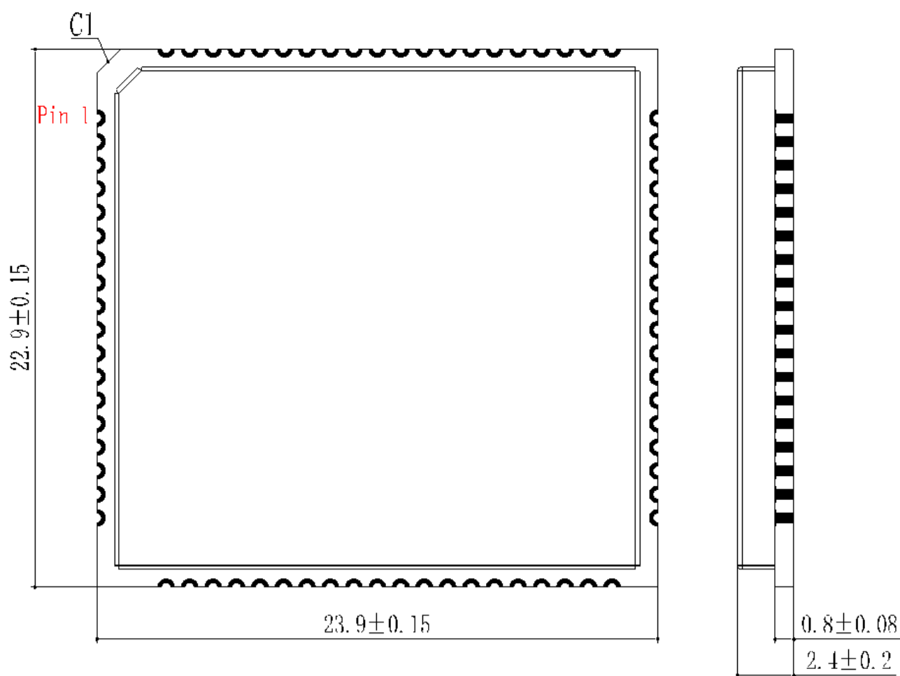
图 42：俯视及侧视尺寸图
