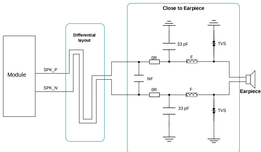
图 29：听筒接口参考电路
