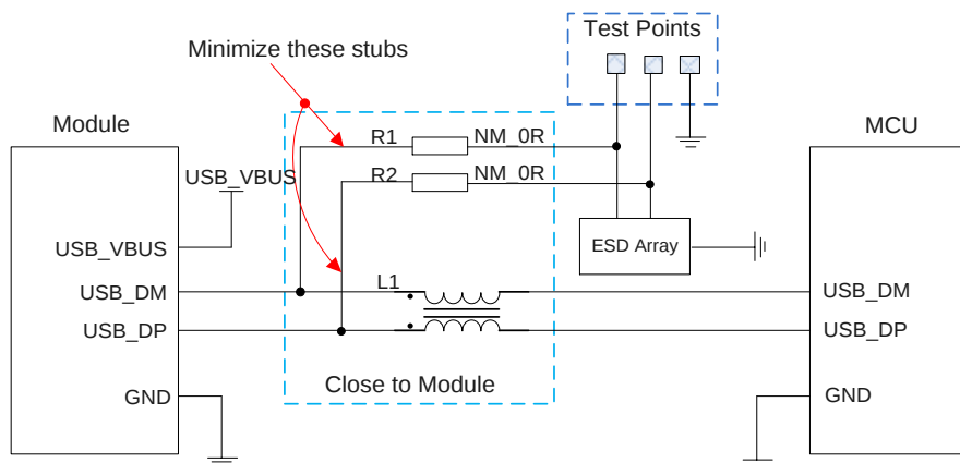
图 22: USB 接口参考设计
