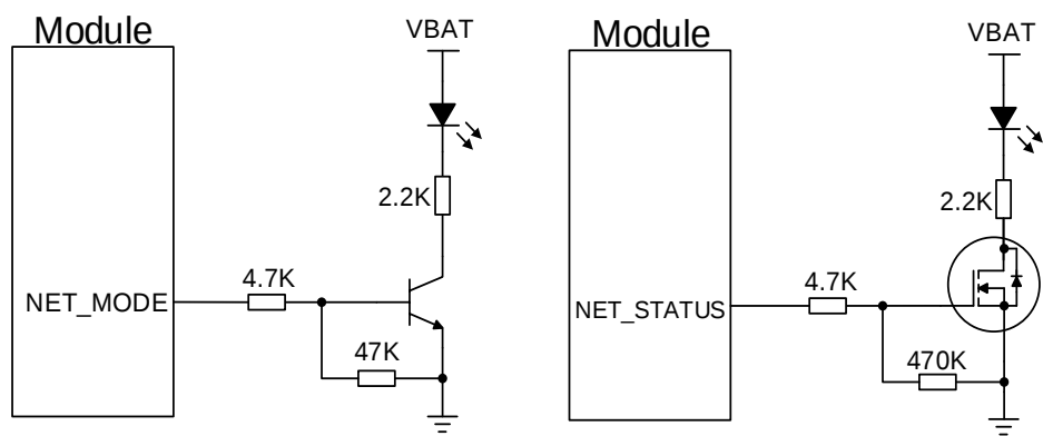
图 32：网络状态指示接口参考电路
