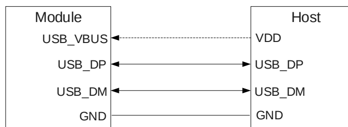
图 5：支持 USB 挂起/唤醒功能的睡眠应用
