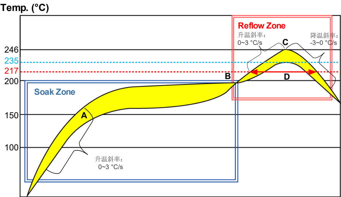
图 46：回流焊温度曲线
