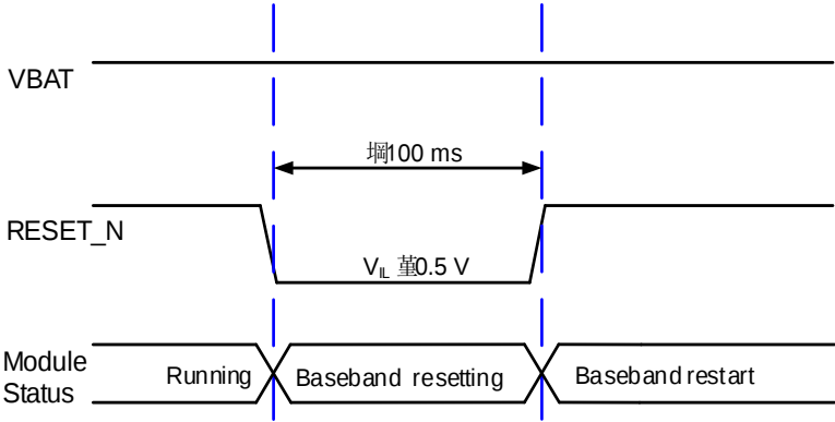
图 19: RESET_N 复位时序图
