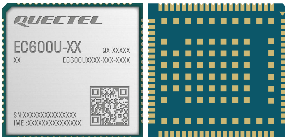
图 45：模块俯视图和底视图
