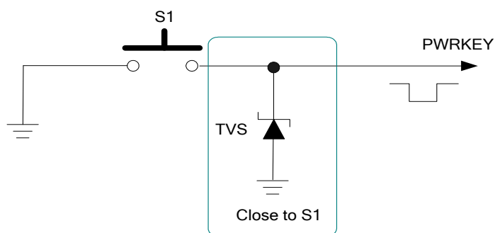
图 14: PWRKEY 按键开机参考电路
