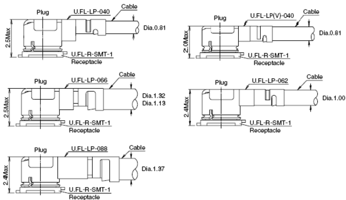
图 41: 射频连接器安装图 (单位: 毫米)
