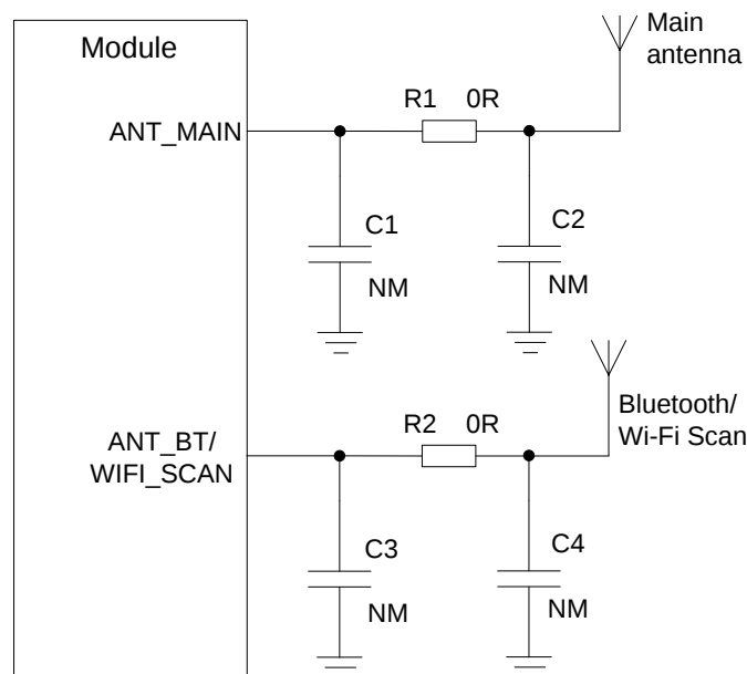
图 34：射频参考电路
