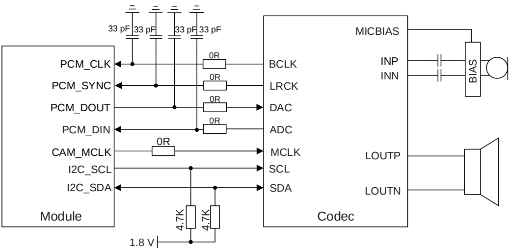
图 26: PCM 和 I2C 接口电路参考设计
