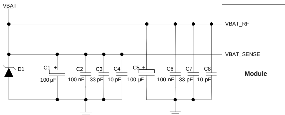
图 9：模块供电电路（不带充电功能）
