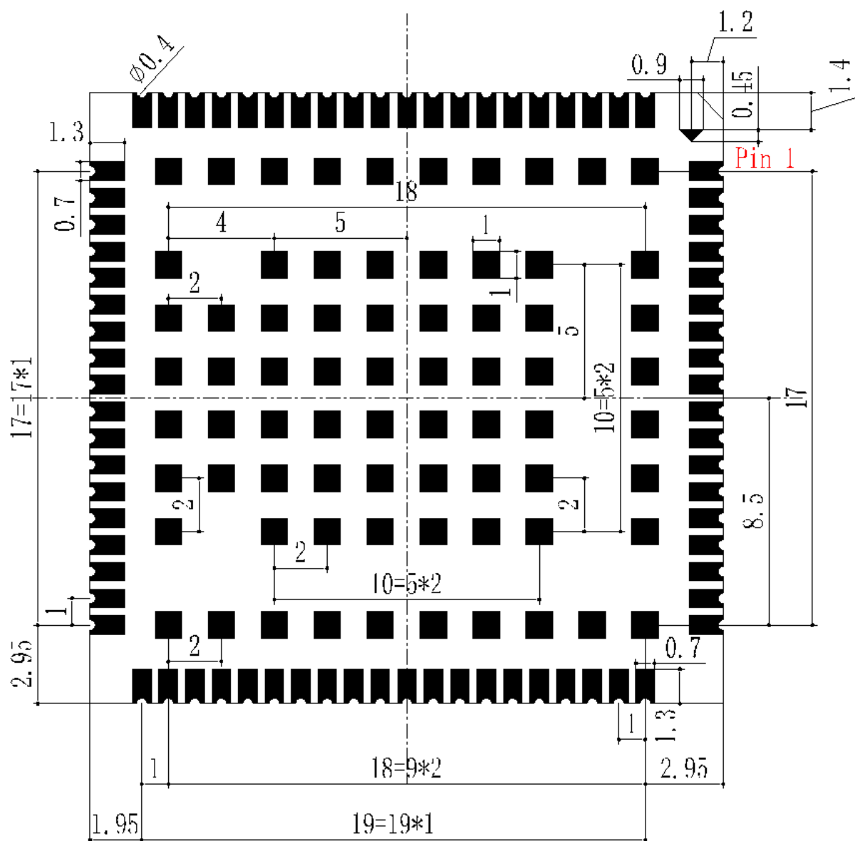
图 43: 底部尺寸图
