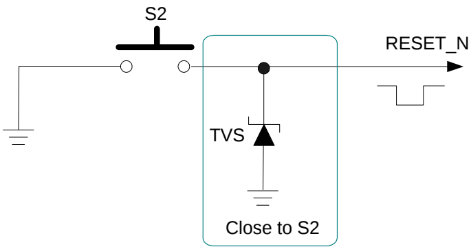
图 18: RESET_N 按键复位参考电路
