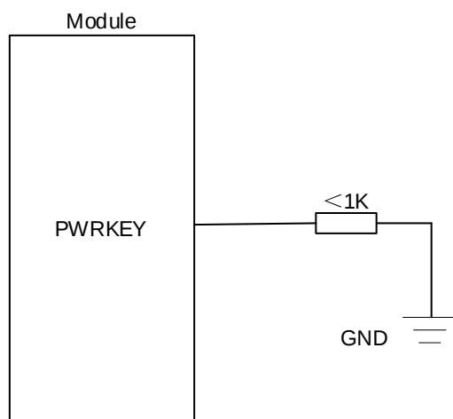
图 13: 上电自动开机参考电路图
