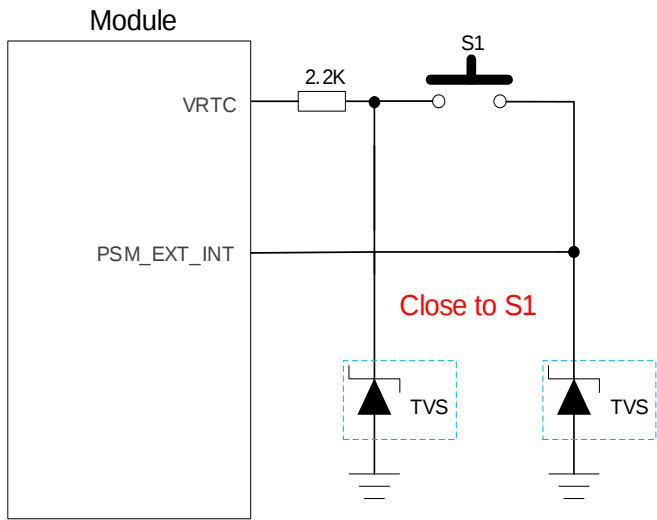
图 7：通过 PSM_EXT_INT 唤醒模块退出 PSM 参考电路
