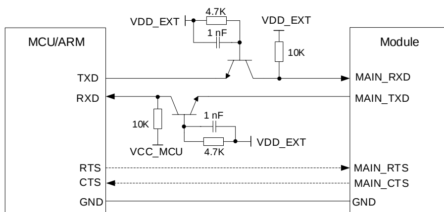
图 24：三极管电平转换参考电路
