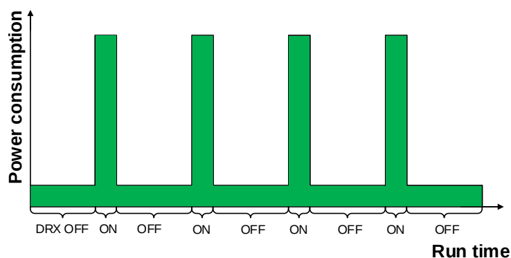
图 3：睡眠模式下模块功耗示意图
