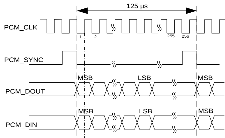
图 25: PCM 时序图
