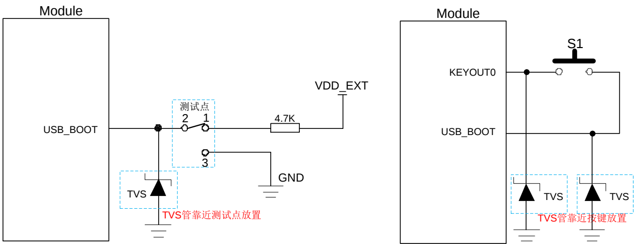
图 33: USB_BOOT 接口参考设计电路
