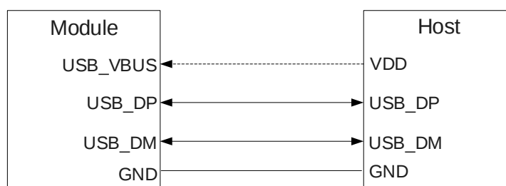
图 4：支持 USB 远程唤醒功能的睡眠应用
