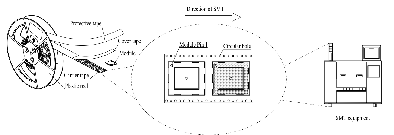
图 49：贴片方向
