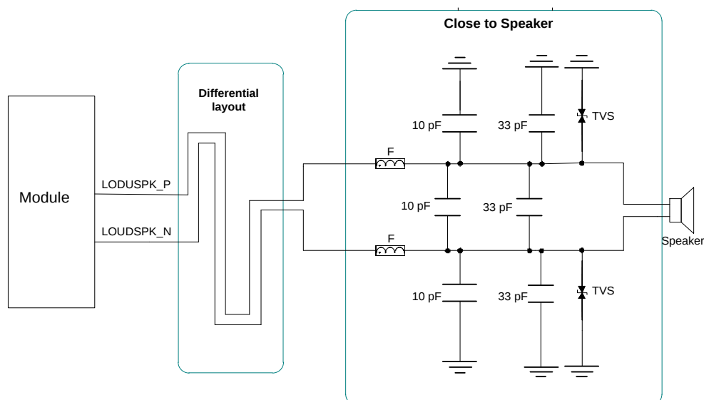
图 28: 扬声器接口参考电路
