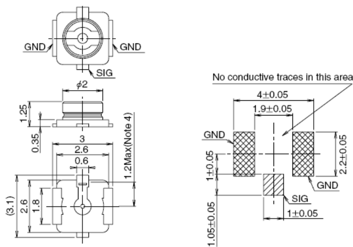
图 39：天线座尺寸（单位：毫米）
