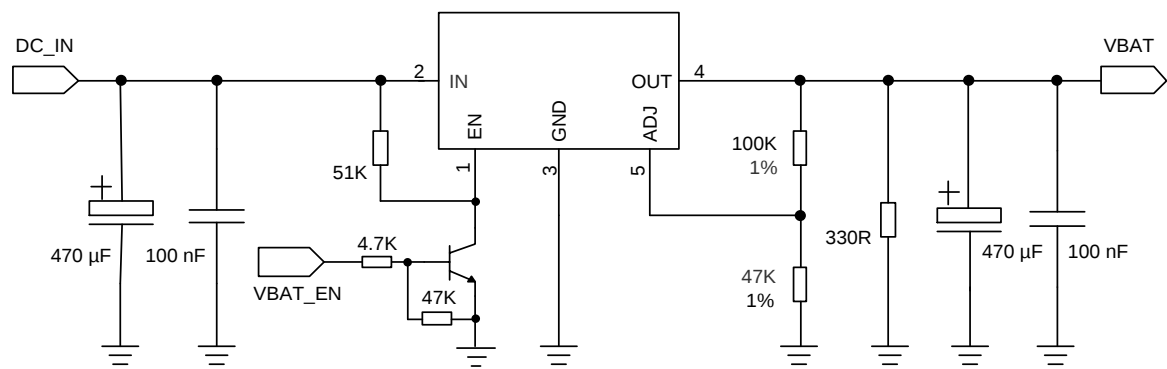
图 11: 供电输入参考设计
