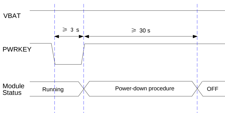
图 16：关机时序图
