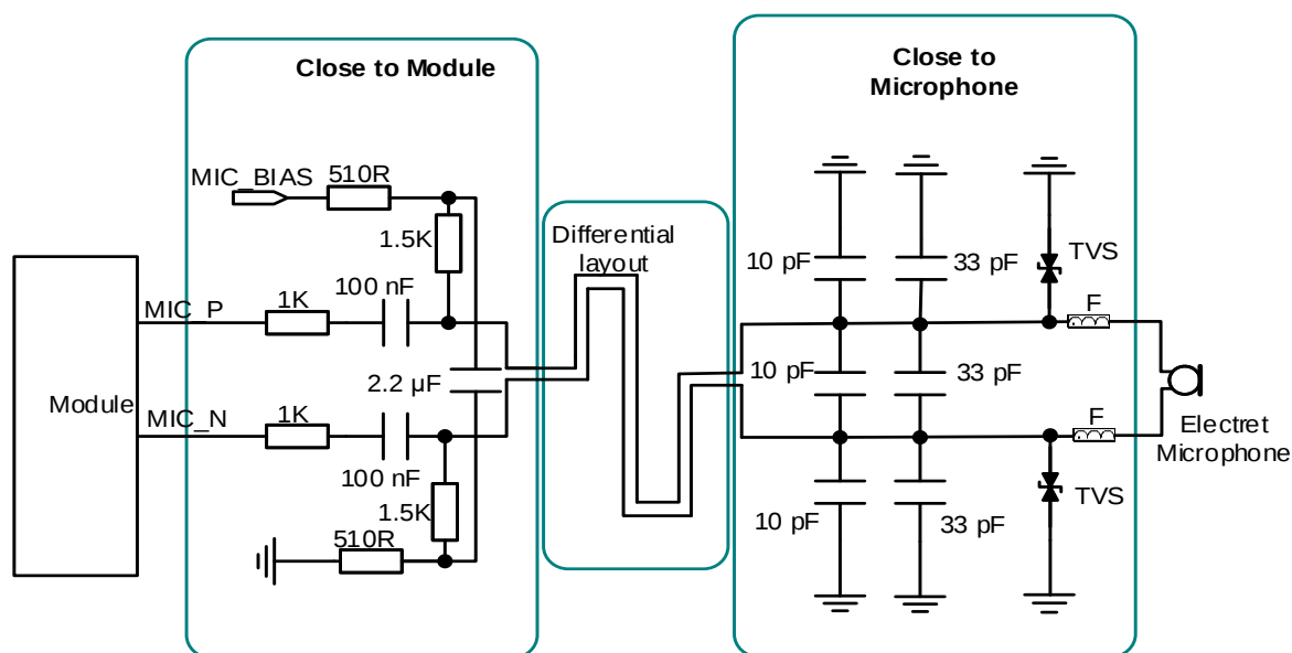
图 27: 麦克风接口参考电路
