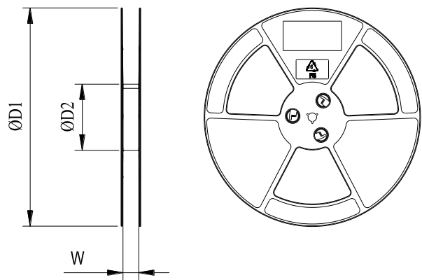
图 48：胶盘尺寸图
