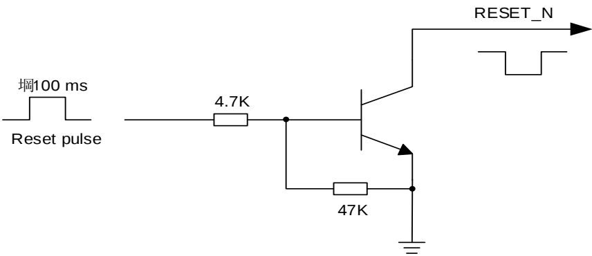
图 17: 开集驱动复位参考电路
